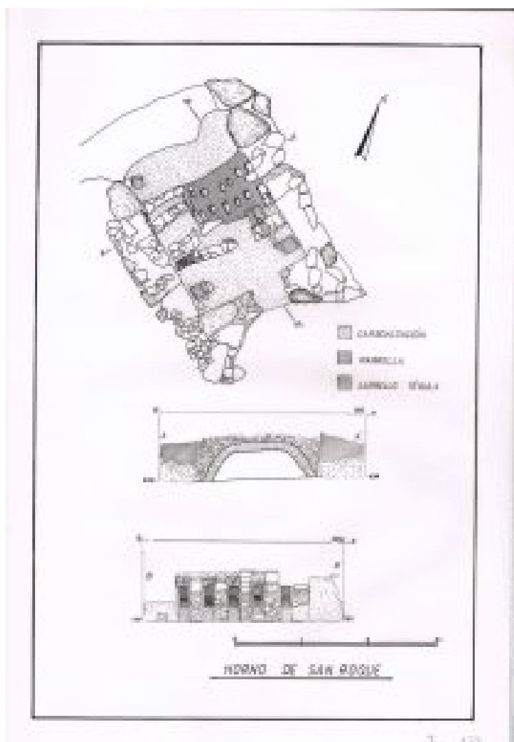
Figura 2. Plano y secciones del horno de Xardín de San Roque (Imagen de Covadonga Carreño Gascón y Enrique González Fernández 1995).
